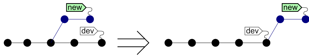
Figure 20. Git Rebase.
